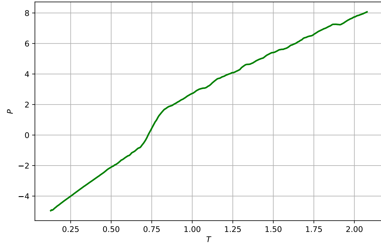
Nyomás - hőmérséklet
