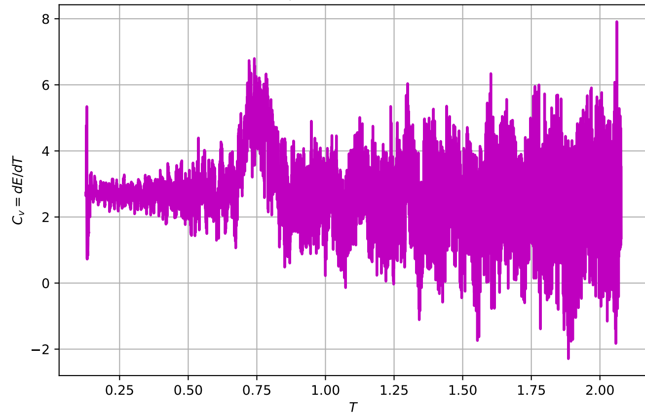
Hőkapacitás - hőmérséklet
